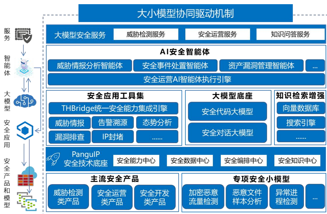
图 11 安星智能安全助手技术架构图
