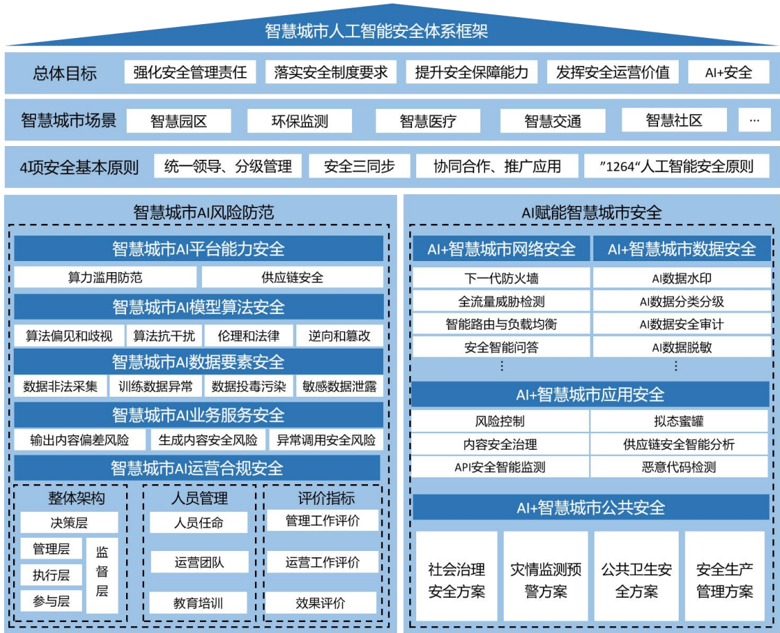
图 3 AI+智慧城市安全解决方案体系框架
