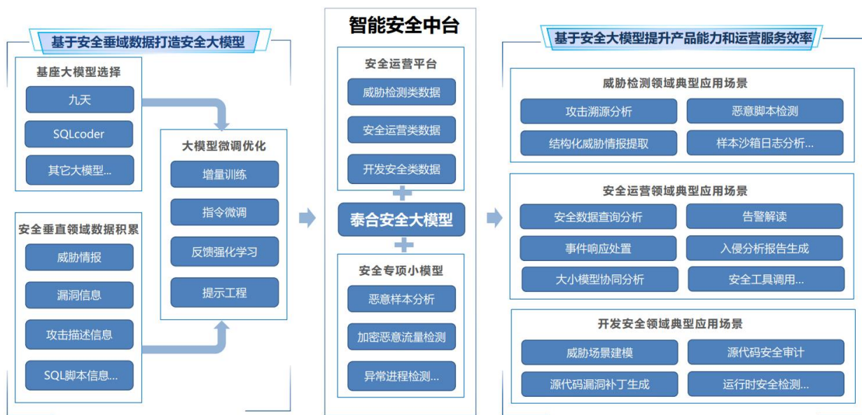
图 10 安星智能安全助手技术应用路线
